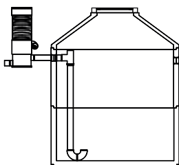
Wirbelfeinfilter eingebaut
